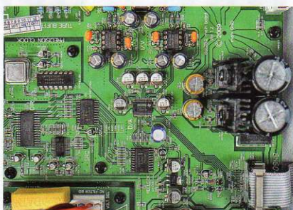
Przetwornik Burr-Browna z układem upsamplera.
