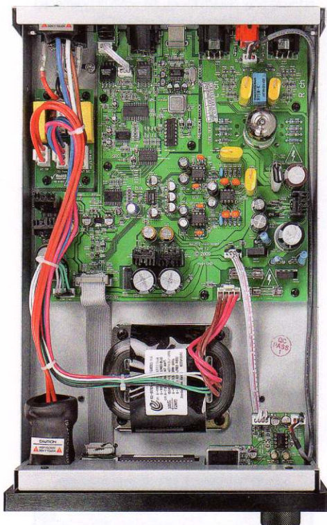
Z przodu trafia R-core, za nim płytka, na której widać lampkę na wyjściu.
